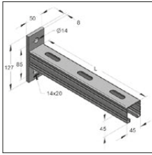
Konsola gotowa 45/45/2,0 mm
